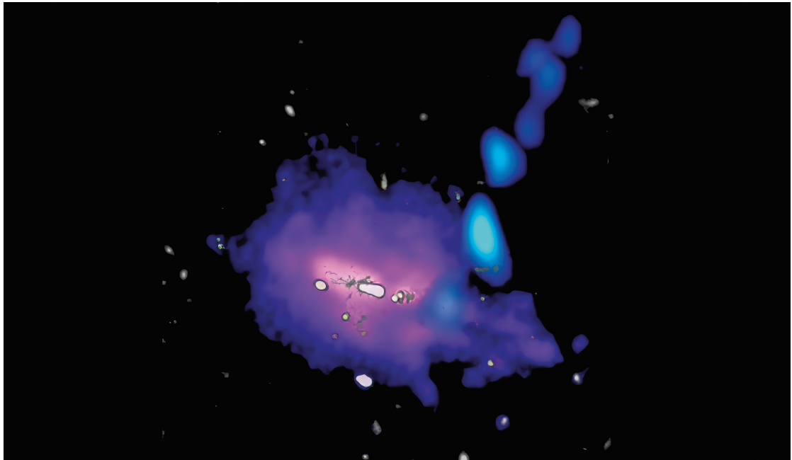
B. Emonts/NRAO/AUI/NSF
