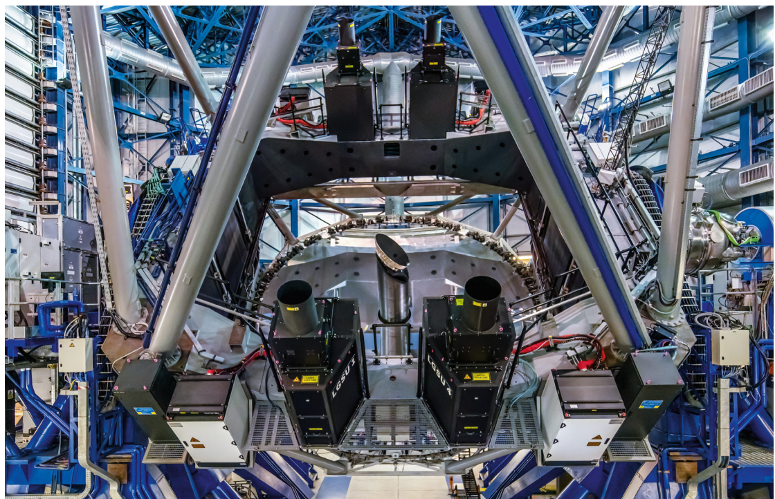
Zdenek Bardon/ESO
